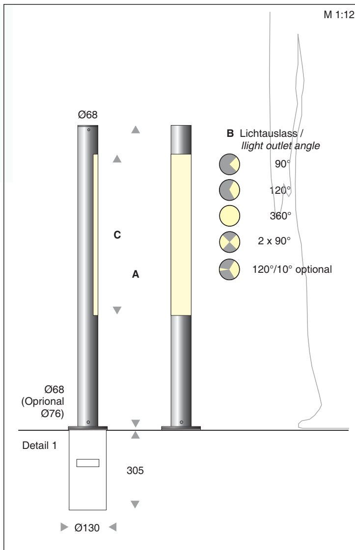
Optional Lichtschlitz rückseitig / light slit on back
