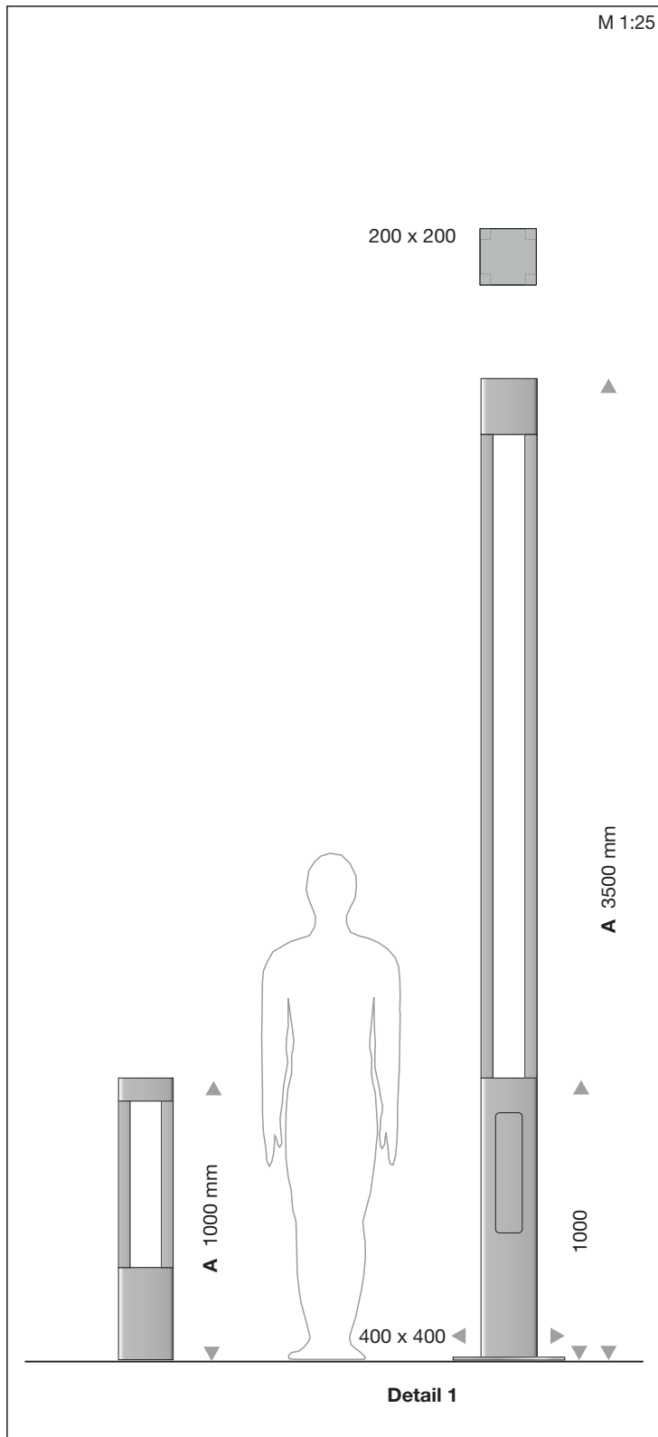
Detail 1 Optional Köcherfundament - siehe Seite 1.14 sleeve foundation - see page 1.14
